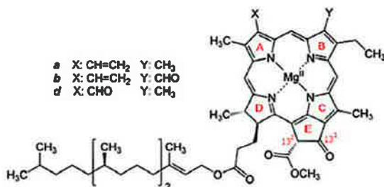
Abb. 10: Strukturformel Chlorophyll.
